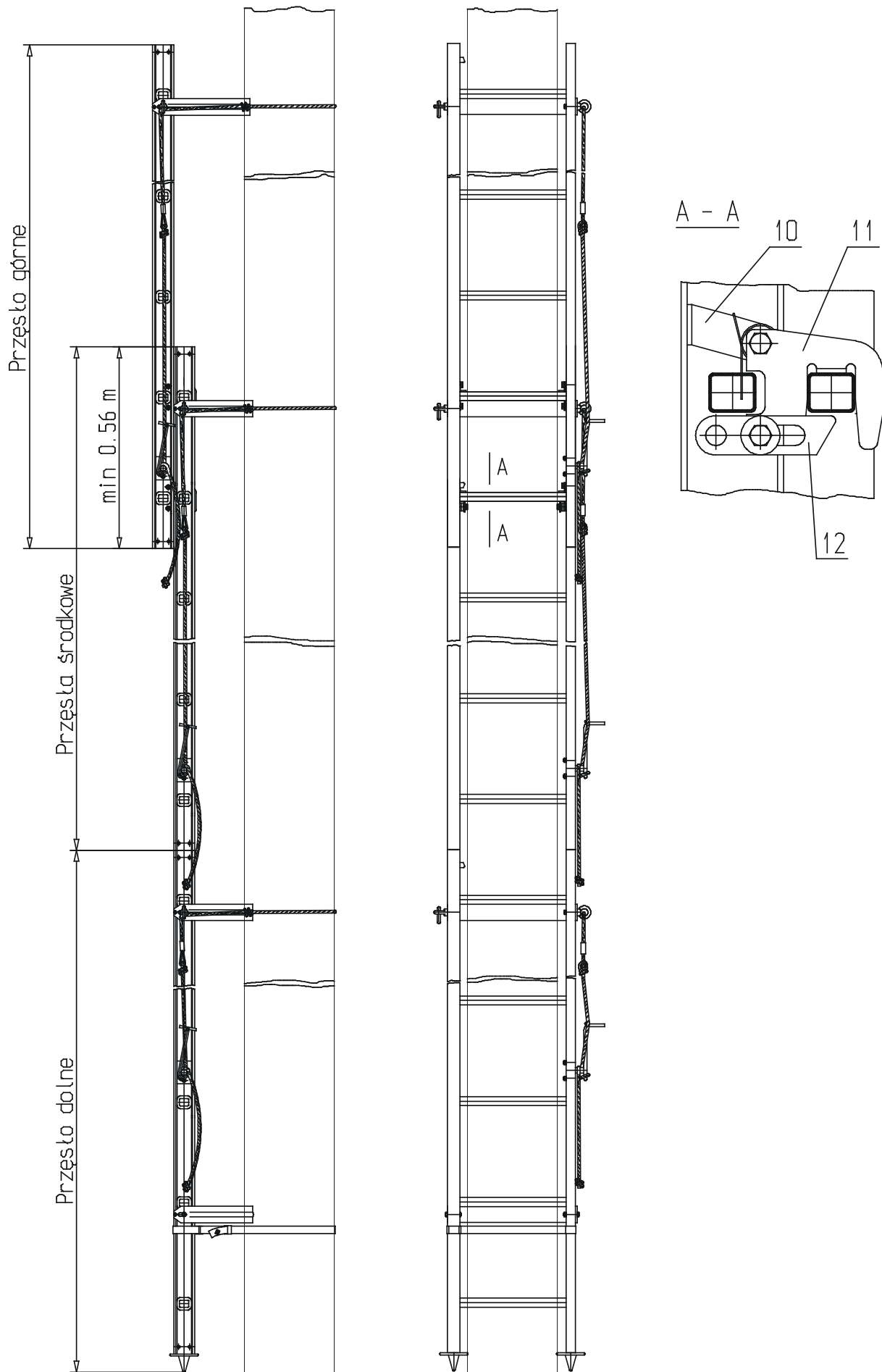
Rys.5. Regulacja wysokości drabiny DRN-22 nasadzonym przęselem górnym
