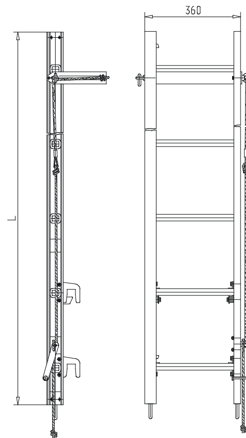
Przęsło górne
