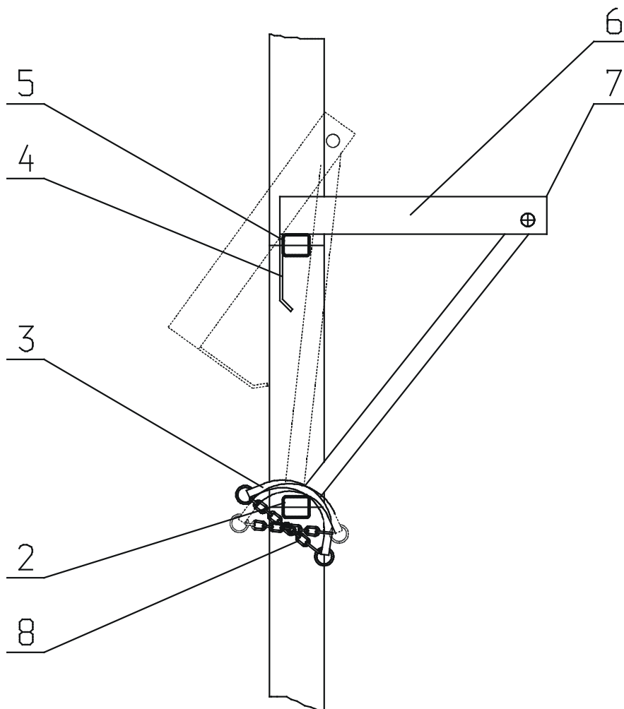
Rys.7. Podest
