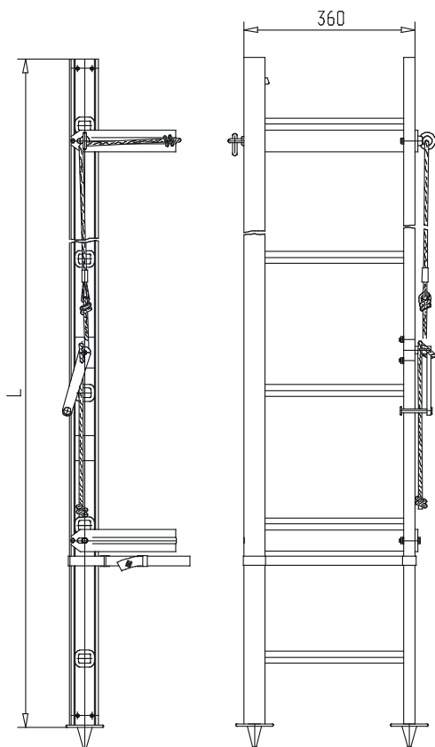
Przęsło dolne
